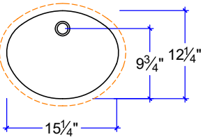
CS-1512* 15 1/4" x 12 1/4" x 5 3/4" 2 molds
