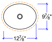
CS-1310^A 12 7/8" x 9 7/8" x 4 1/2" ♿
