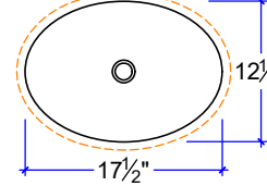
CS-1712* 17 1/2" x 12 1/2" x 5 3/4" 2 molds
