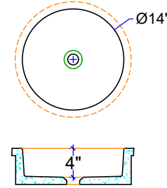
CS-14D-FB ♿ 14" DIA. x 4" DEEP
