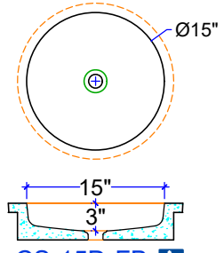
CS-15D-FB ♿ 15" DIA. x 3" DEEP 5 Molds
