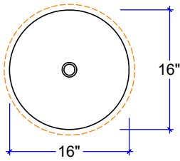
CS-16D* 16" DIA. x 8" DEEP 4 molds
