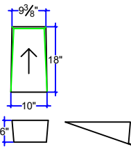
1018-B or 1810-R/L
