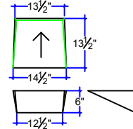
1514-B or 1415-R/L
