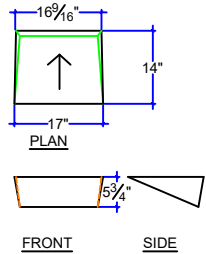
1714-B or 1417-R/L (5)
