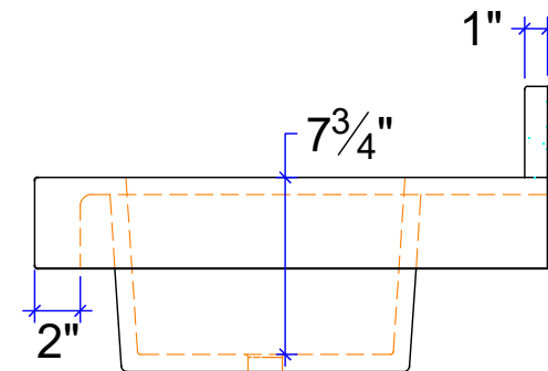
RIGHT ELEVATION
